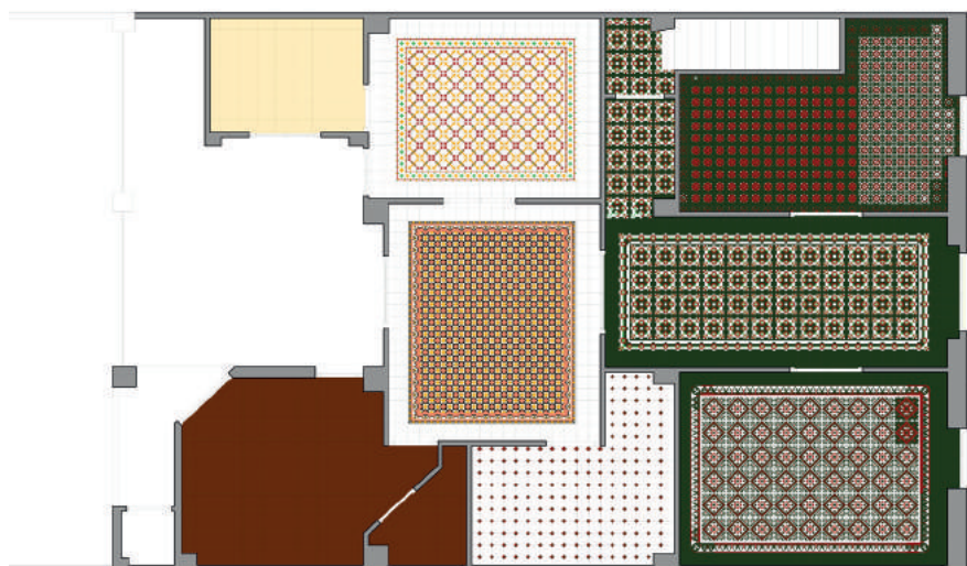
Planta superior
