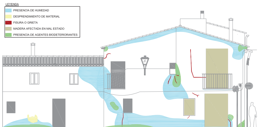
Fachada calle Mossén Rausell
