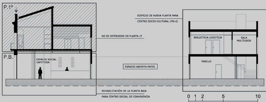
Sección
