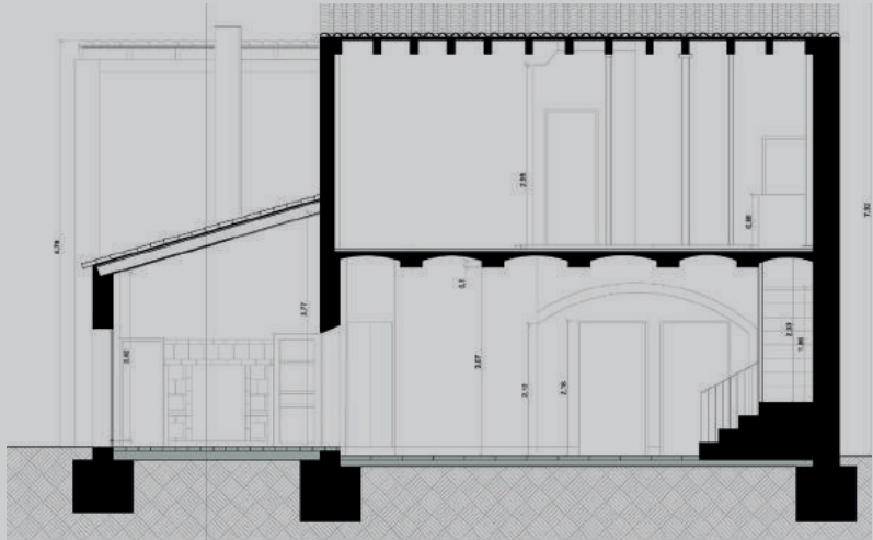
Sección longitudinal
