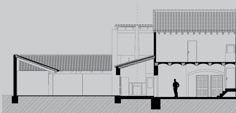
Secciones
