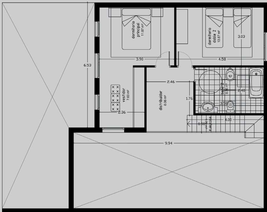
Planta superior
