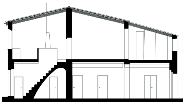
Secciones
