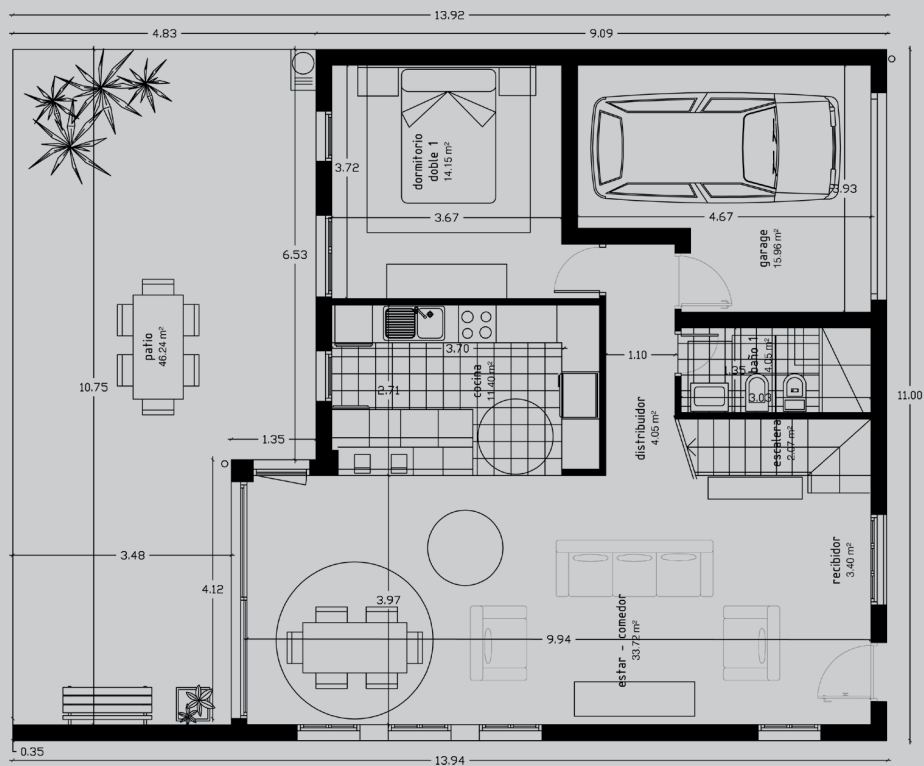
Planta baja
