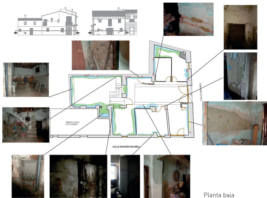
Planta baja
