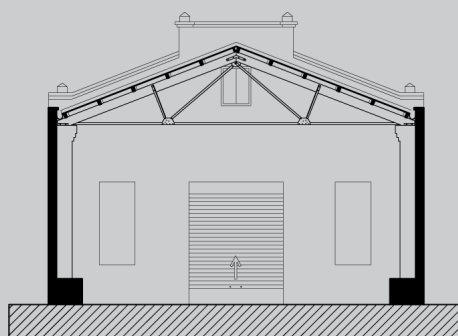
Sección D-D'
