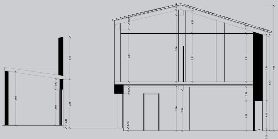
Sección C-C'
