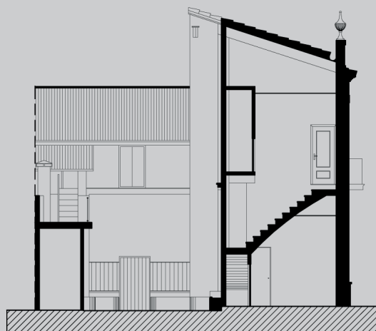
Sección C-C'
