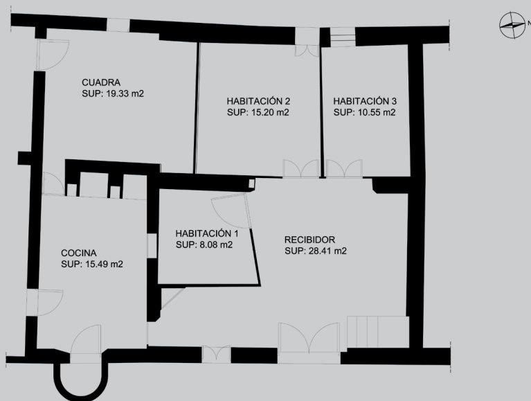
Planta baja
