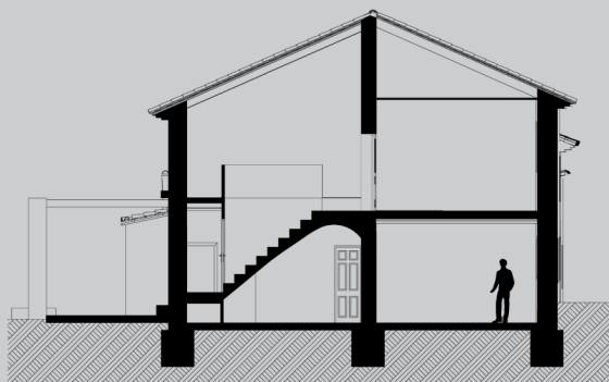
Secciones
